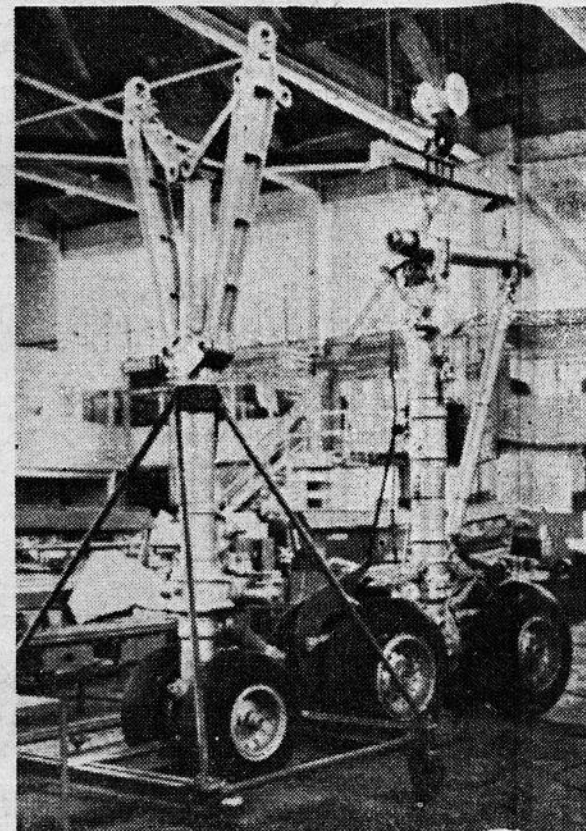
Le train principal de « Concorde » étudié et construit par Hispano-Suiza.
