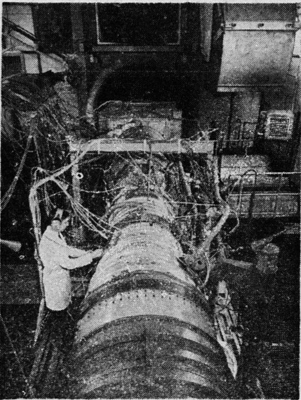
SNECMA. Centre de Villaroche. Installation d'un Olympus 593 dans le banc d'essai spécialement construit pour ce type de réacteur.
